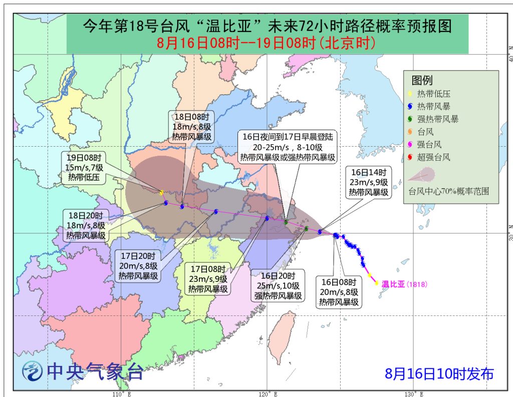
台风“温比亚” 8月16日10时路径预报图
